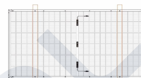
Vnější čtyřotvorová montáž šroubem, nosník kolmý k dlouhému rámu
