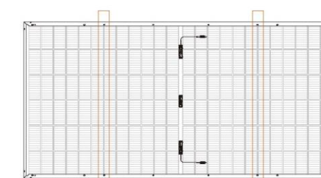
Vnitřní čtyřotvorová montáž šroubem, nosník kolmý k dlouhému rámu
