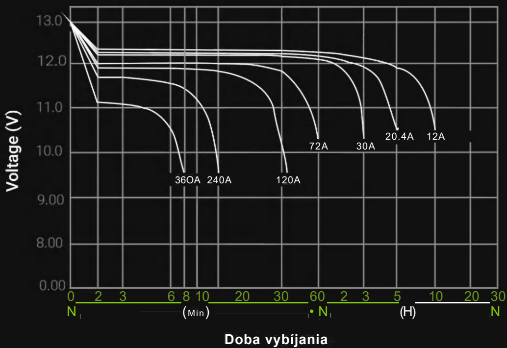
Vybíjacia charakteristika po plnom nabití (25°C, 77°F):
