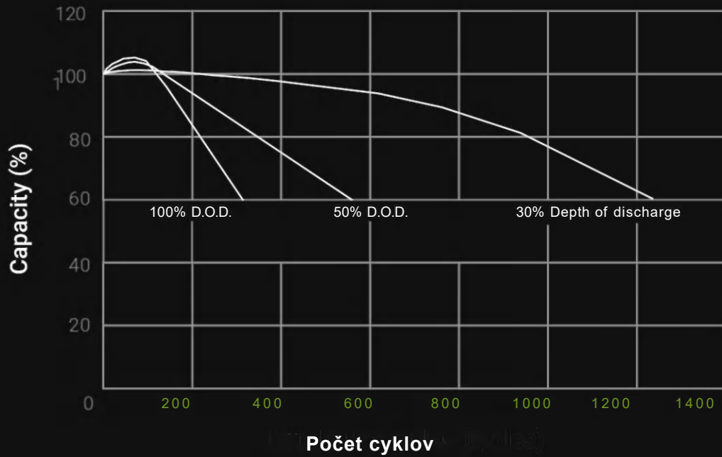
Cyklická životnosť v závislosti od hĺbky vybitia (DOD)
