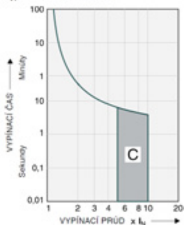
Vypínacia charakteristika C
