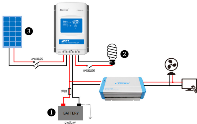
Obrázek 2-2 Schéma zapojení
