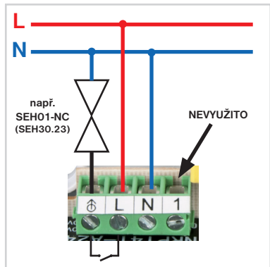
Obr.3 Zapojte přírodní vodiče podle schématu.
